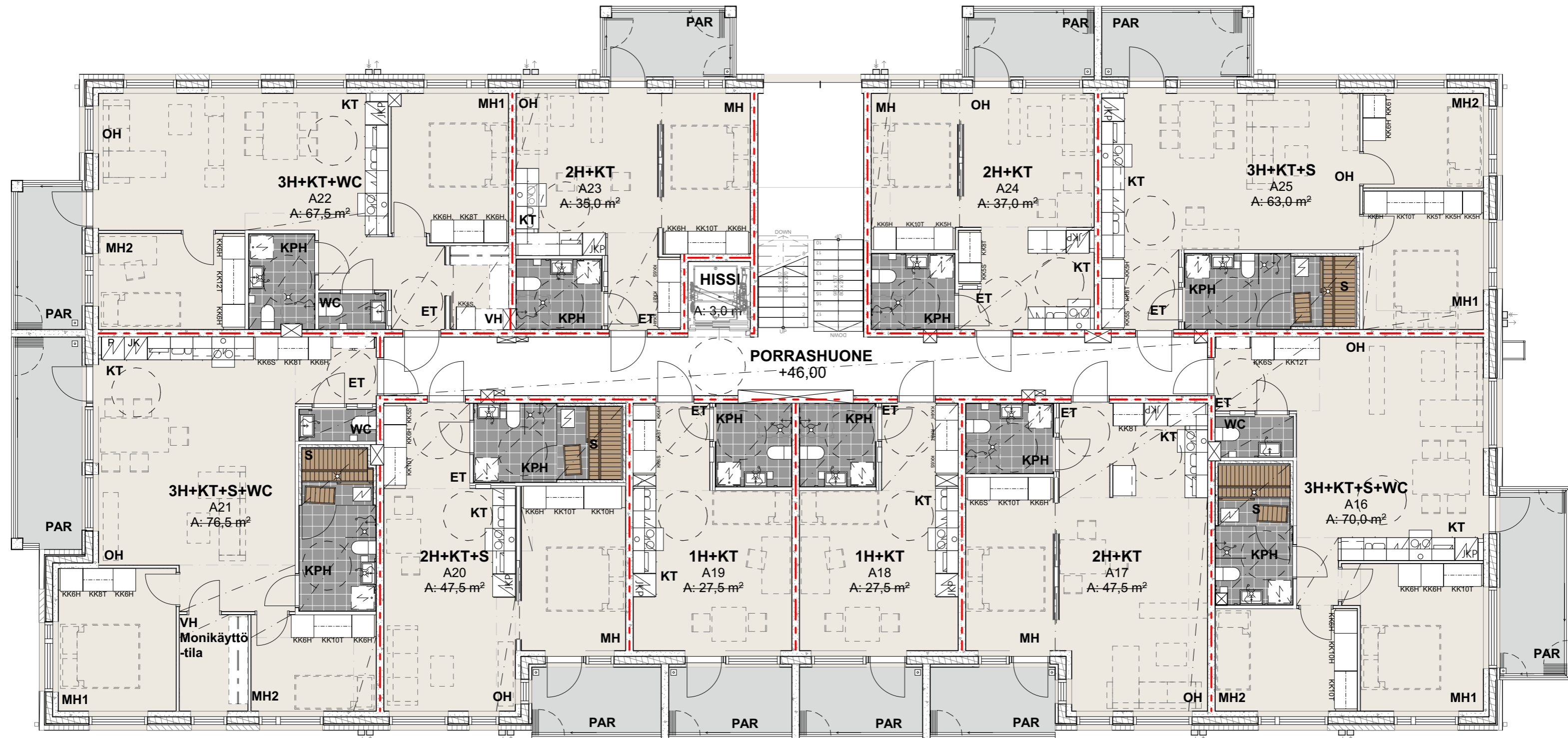
3.krs MITTAKAAVA: 1:100
