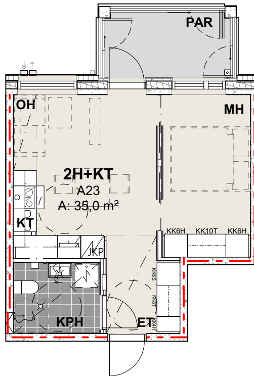
2H+KT 35.0 m 2 MITTAKAAVA: 1:100
